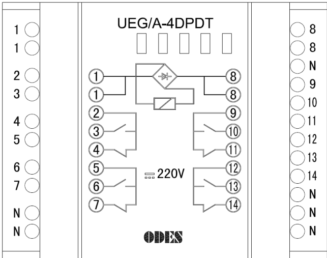
UEG/A-4DPDT
