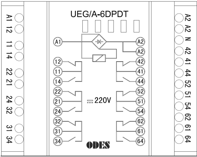
UEG/A-6DPDT
